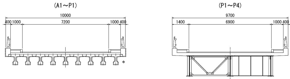
標準断面図
