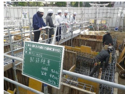
配筋検査
