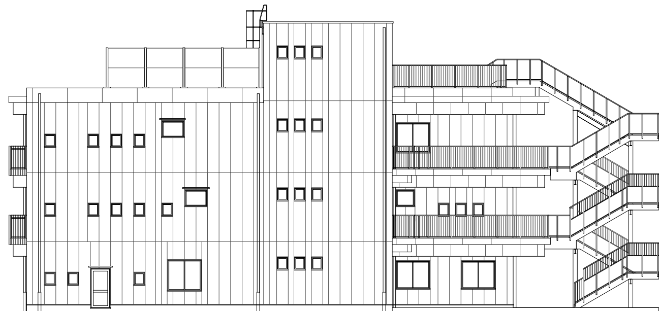
西側立面図
